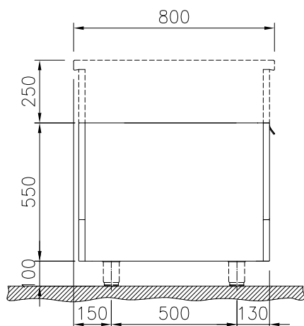
Boven aanzicht
